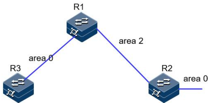
图 3-44 配置 OSPFV3 虚连接的组网图
