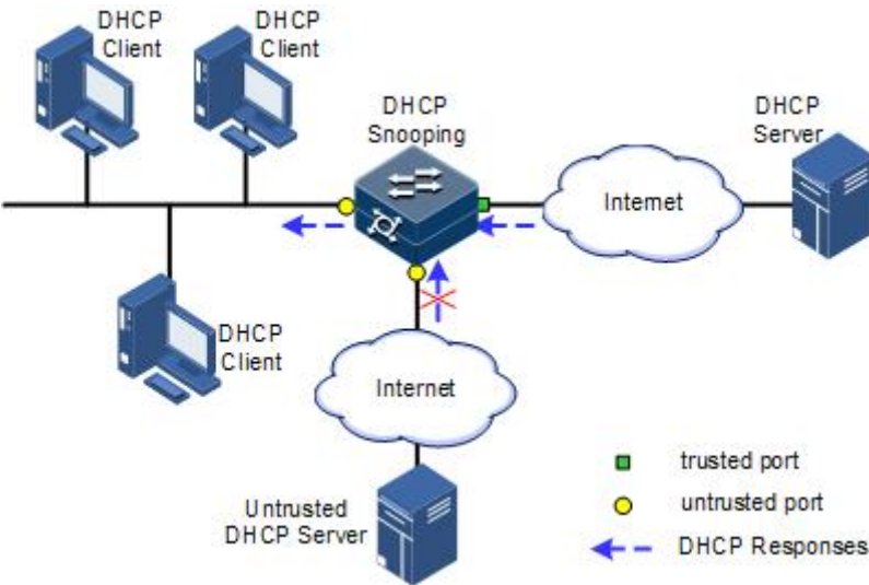
图 8-11 DHCP Snooping 组网示意图
