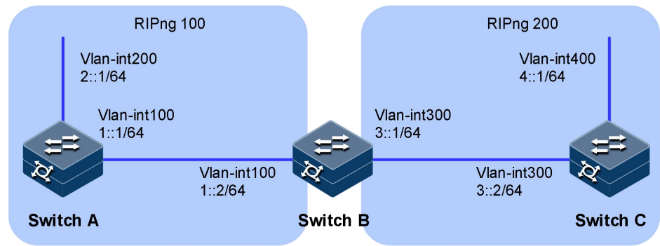
图 3-50 RIPng 引入外部路由组网图
