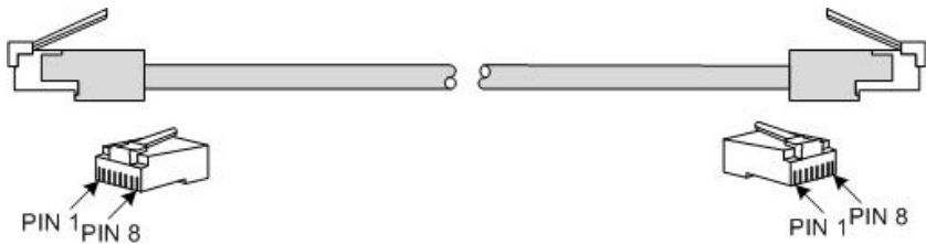
图 3-2 网线示意图
