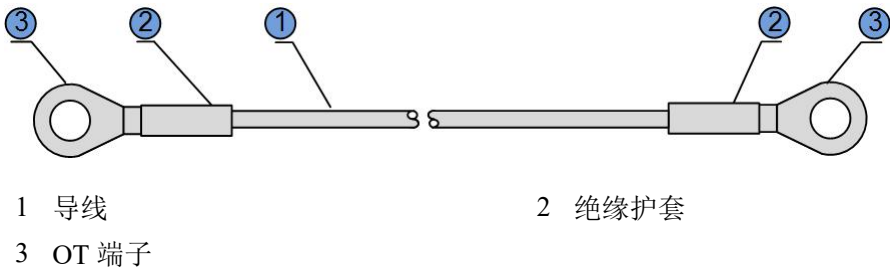
图 3-3 接地线缆示意图
