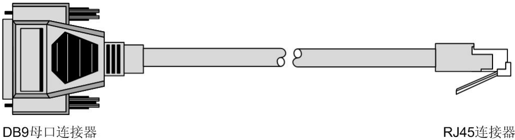
图 2-19 Console 线示意图
