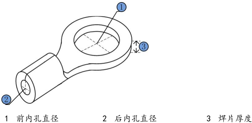
图 2-13 OT 端子示意图
