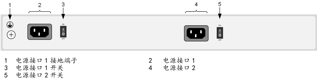
图 2-2 S2700 后面板外观
