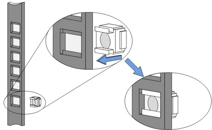
图 4-3 安装浮动螺母
