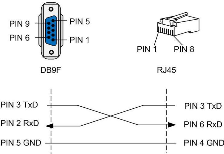
图 2-20 接线关系示意图
