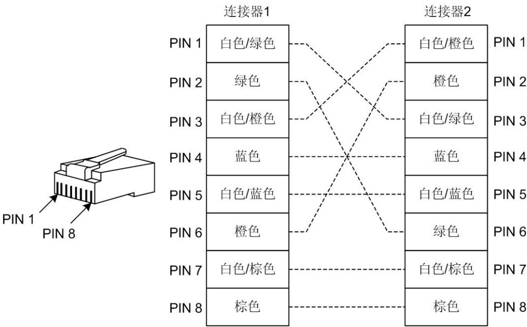
图 2-10 100Mbit/s 交叉网线接线图
