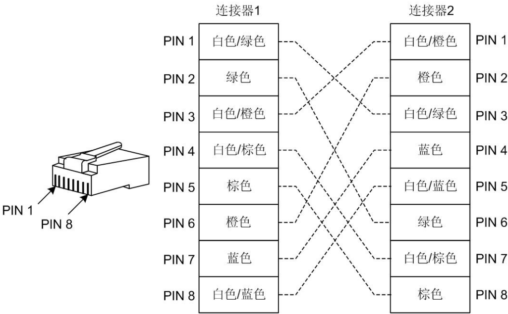
图 2-11 1000M 交叉网线接线图
