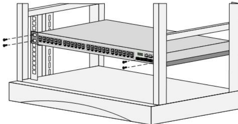
图 4-5 水平安装设备到机架
