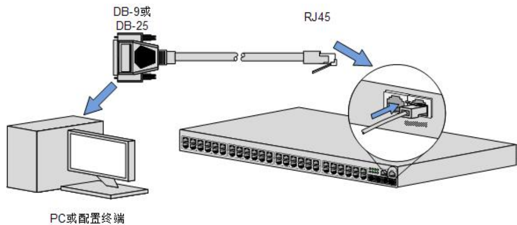
图 4-14 连接 Console 串口线
