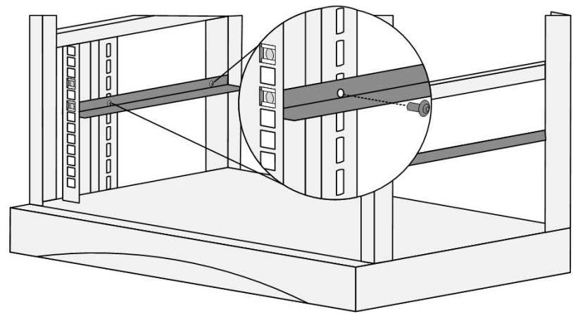
图 4-4 安装滑道
