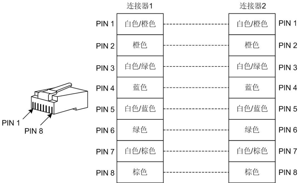
图 2-9 10/100/1000M 直通网线接线图
