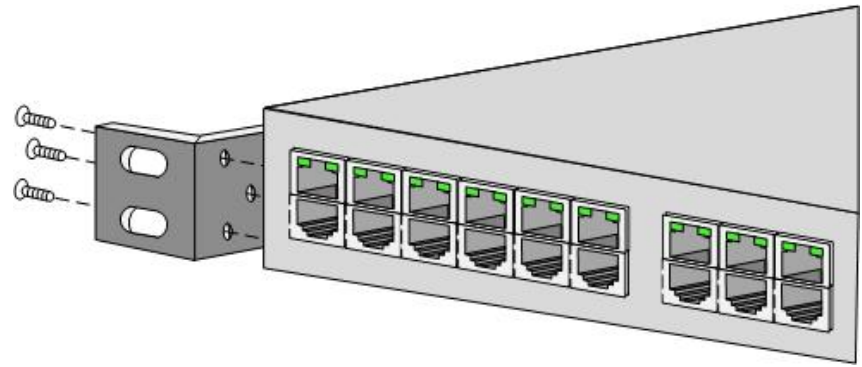
图 4-2 安装挂耳
