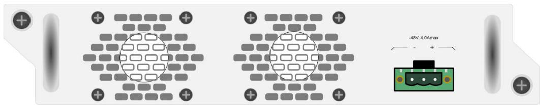
图 2-8 可插拔直流电源模块
