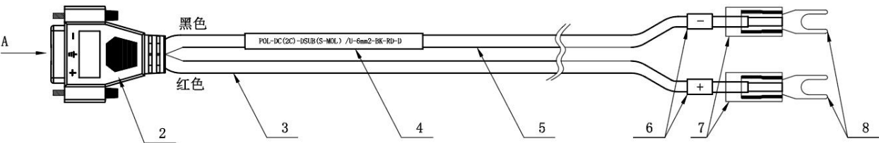
图 2-22 可插拔直流电源线示意图
