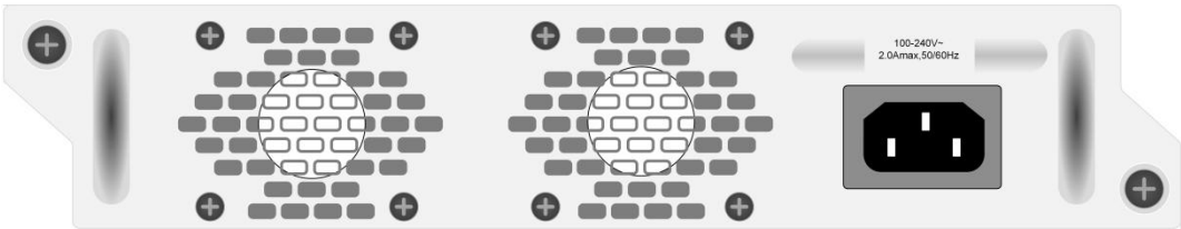
图 2-10 可插拔交流电源模块
