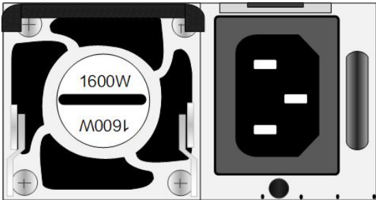
图 2-11 PoE 款型可插拔交流电源模块
