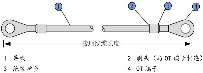
图 2-18 接地线缆示意图
