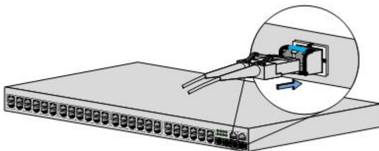
图 4-7 连接光纤
