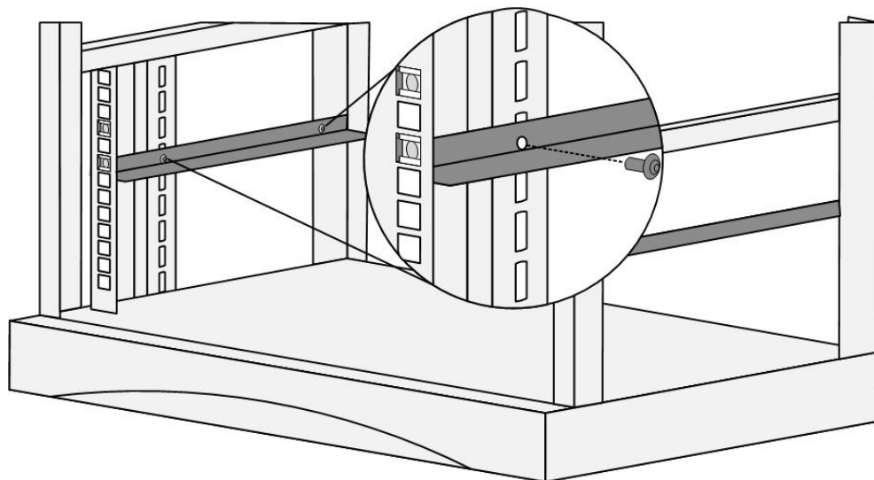
图 4-4 安装滑道
