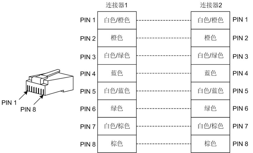
图 2-15 10/100/1000M 直通网线接线图
