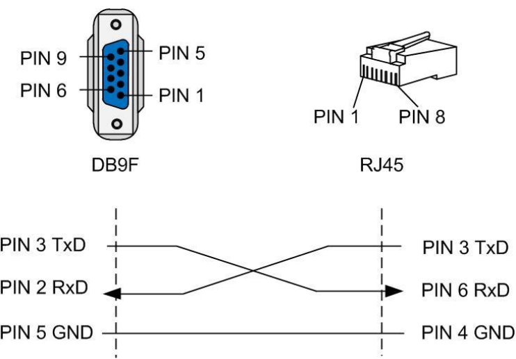
图 2-27 接线关系示意图
