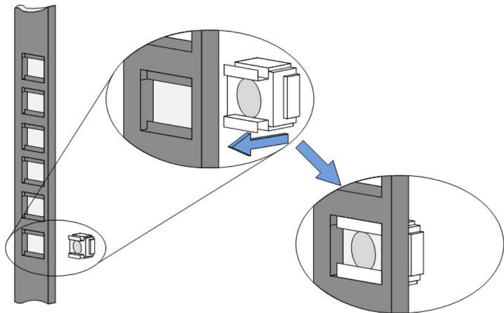
图 4-3 安装浮动螺母
