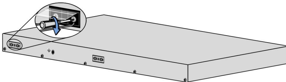
图 4-11 连接直流电源线
