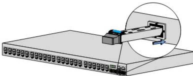
图 4-6 插入 SFP 光模块
