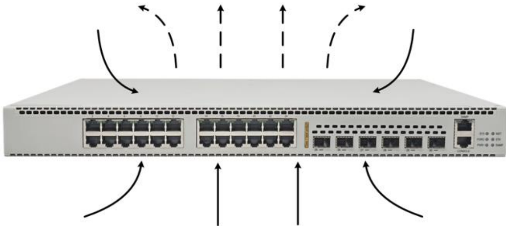
图 2-31 风扇 2 流向示意图
