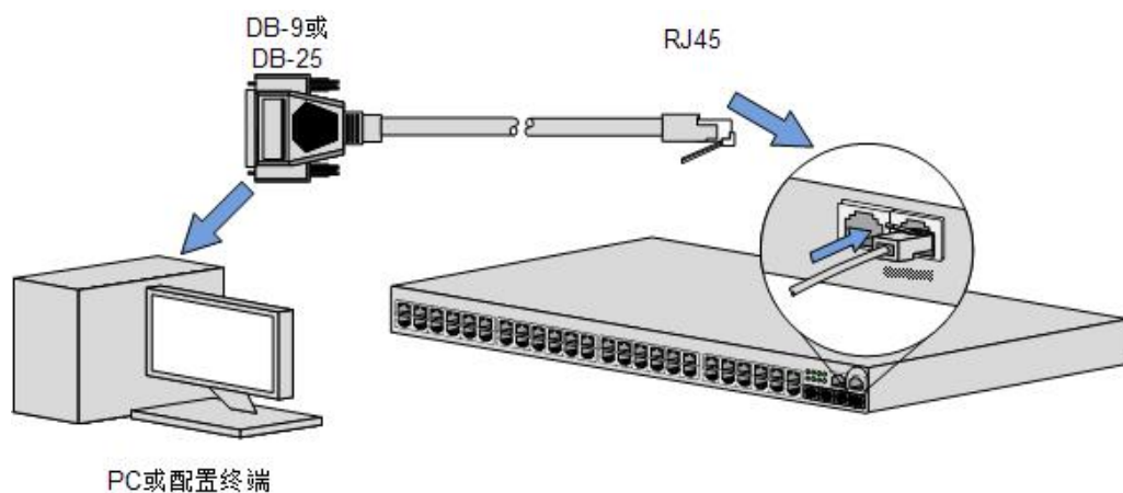
图 4-16 连接 Console 串口线
