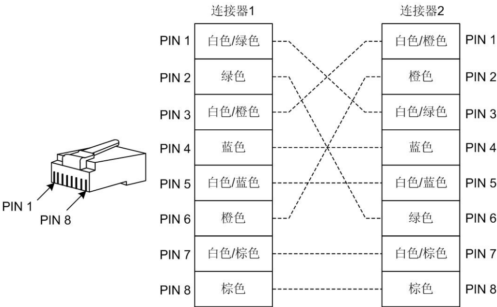
图 2-16 100Mbit/s 交叉网线接线图
