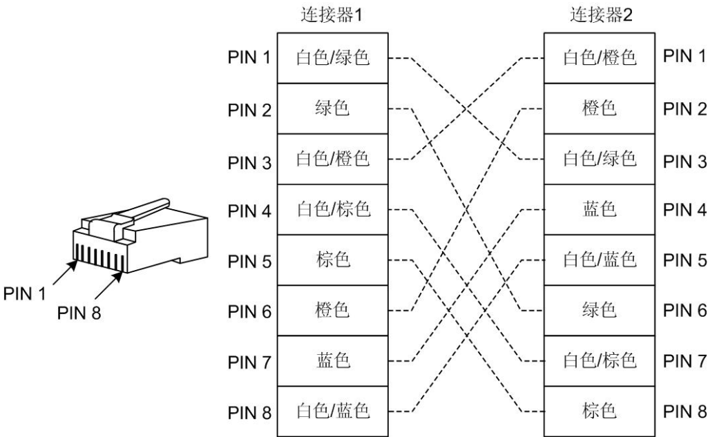
图 2-17 1000M 交叉网线接线图
