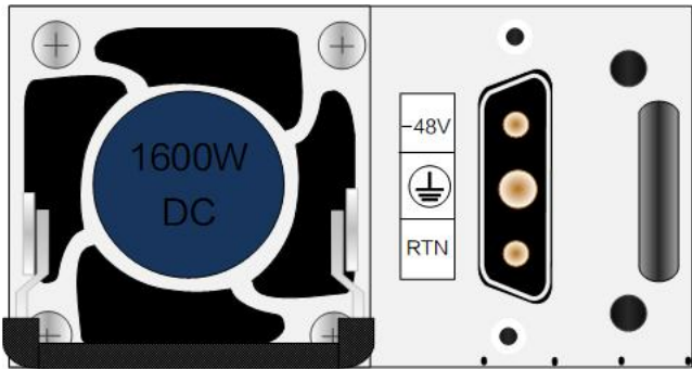
图 2-12 PoE 款型可插拔直流电源模块
