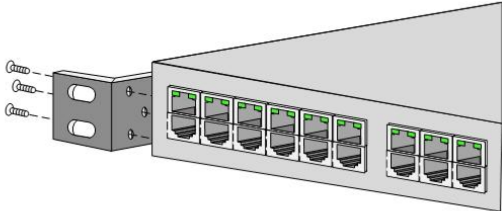
图 4-2 安装挂耳
