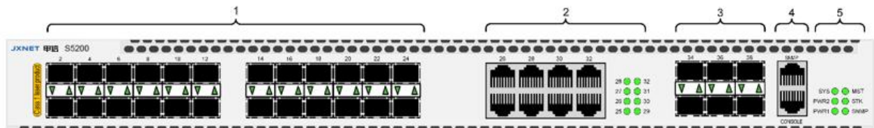
图 2-5 S5200-24S8T6X 前面板外观
