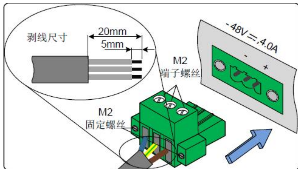
图 4-13 连接可插拔直流电源线缆
