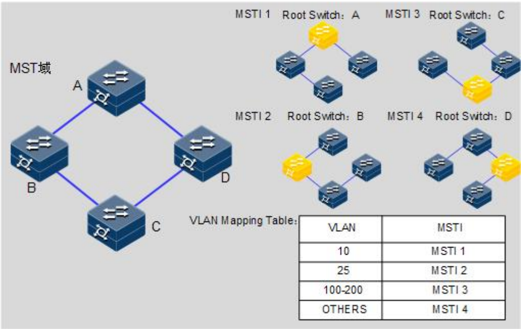
图 1-14 MSTI 概念示意图
