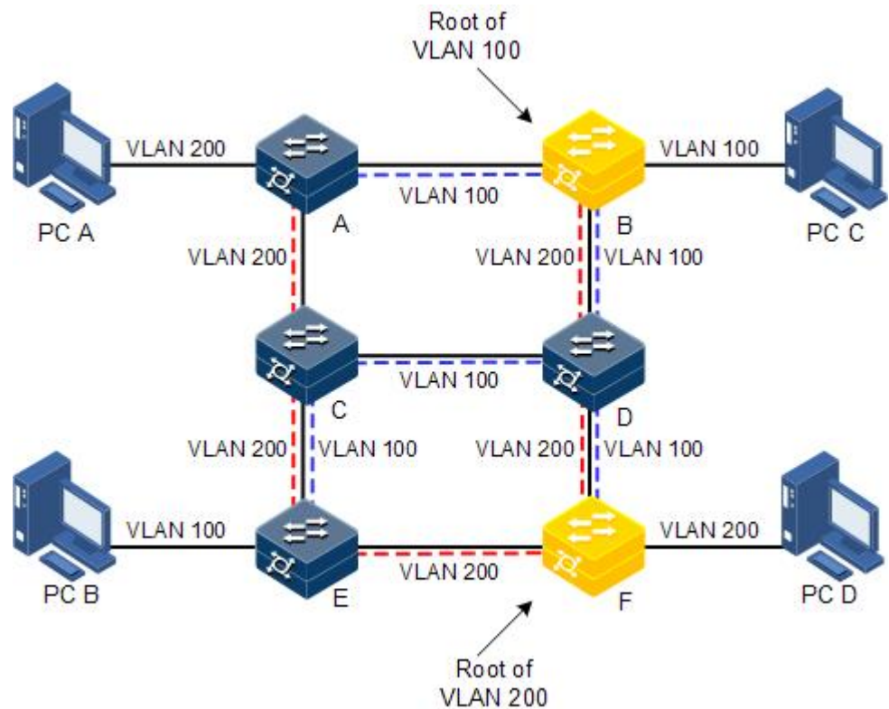
图 1-15 MST 域内多生成树实例组网示意图
