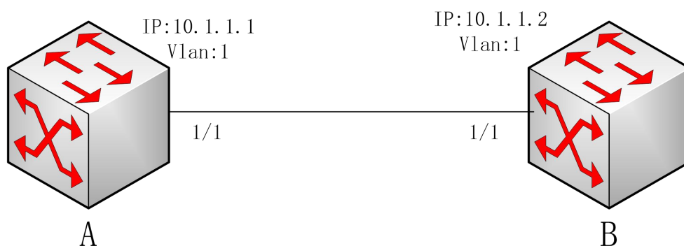
图 1-24 BFD 单跳应用
