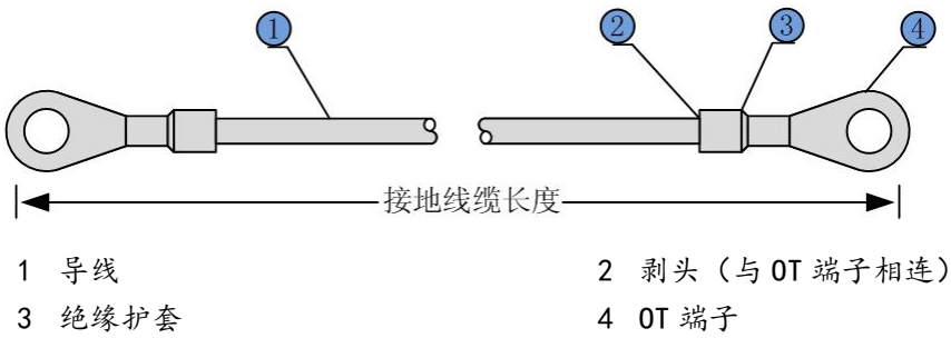
图 2-8 接地线缆示意图
