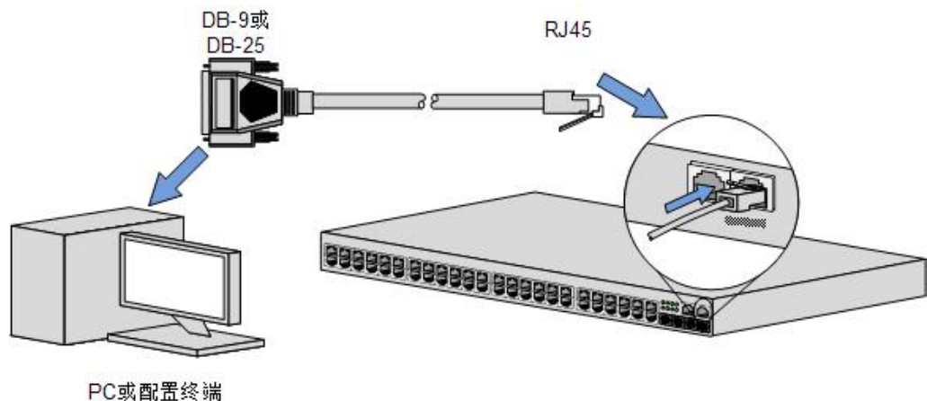
图 4-12 连接 Console 串口线
