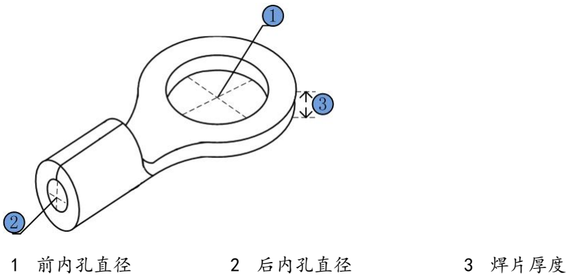
图 2-9 OT 端子示意图
