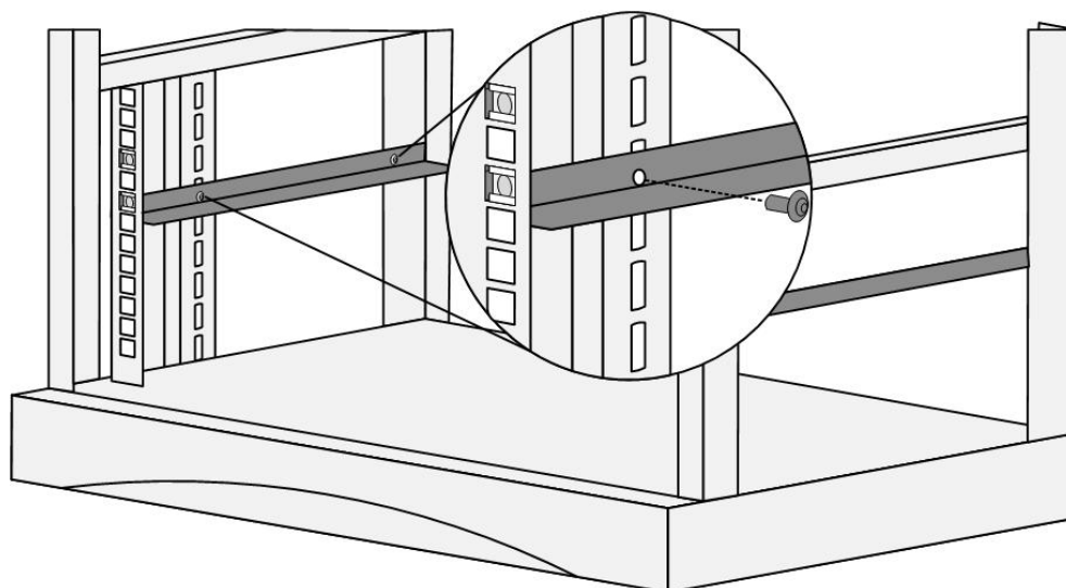
图 4-4 安装滑道
