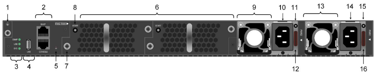
图 2-4 S6600-48X8C 后面板外观
